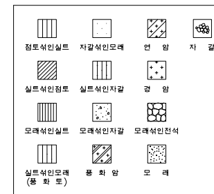
범례종구배도
